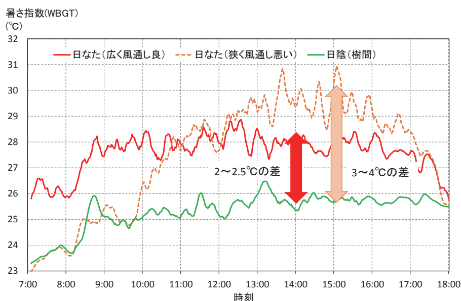
図2-1 日なた(風通しが悪い)及び日陰の暑さ指数(WBGT)の変化
